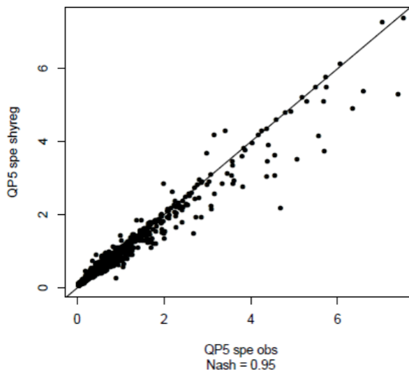
Débits de pointe pseudo-spécifique ( \text{m}^3/\text{s}/(\text{km}^2)^{0.8} ) de période de retour 5 ans observées et simulées
